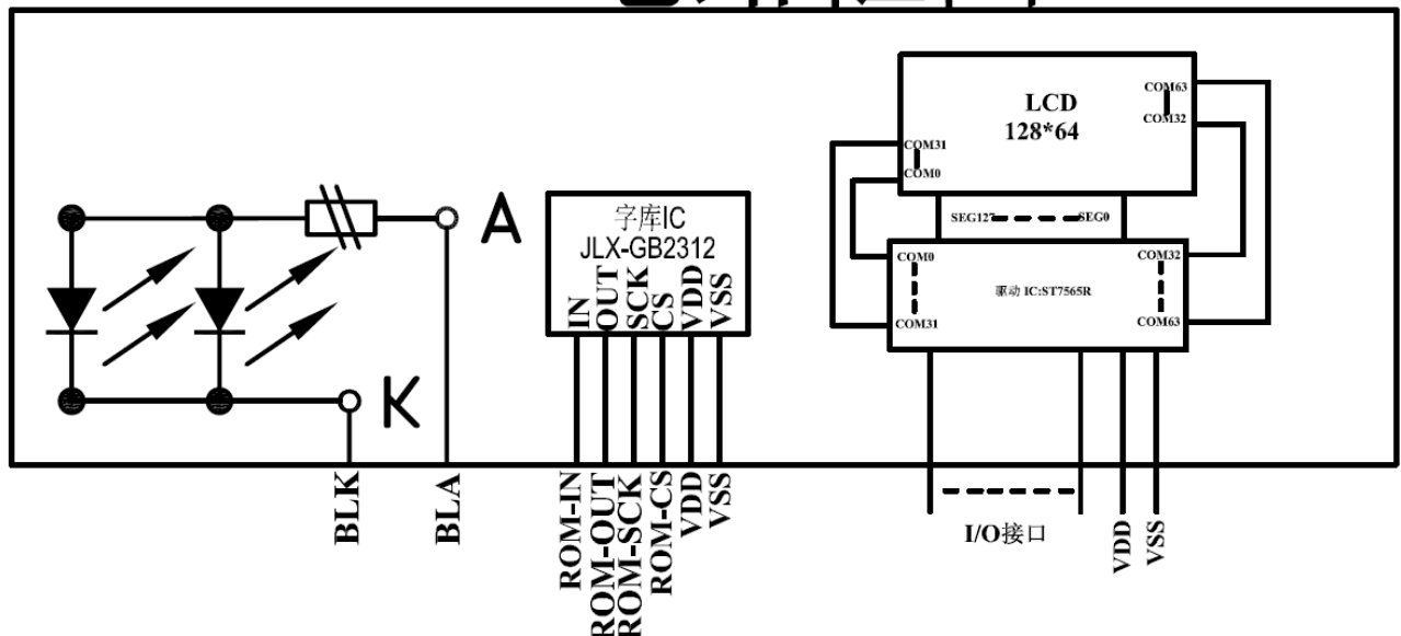
图 2: 电路框图
