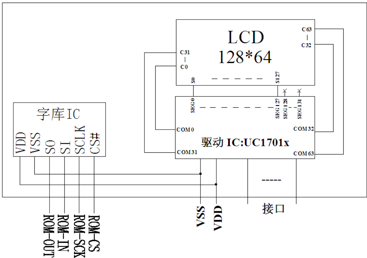
图 2: 电路框图
