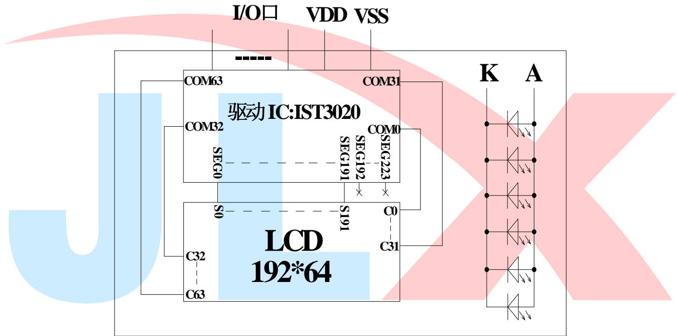
图 2: JLX19264G-329 图像点阵型液晶模块的电路框图
