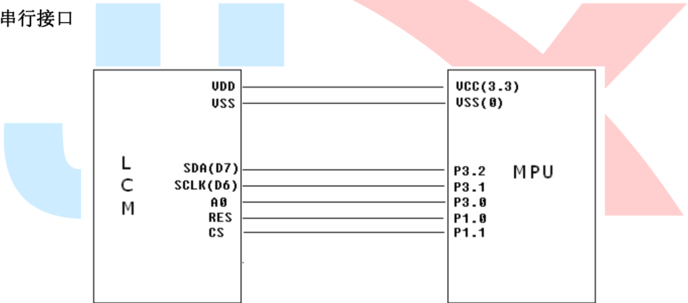
图 9. 串行接口
