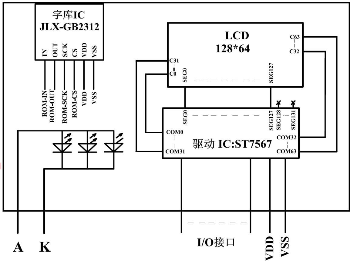
图 2: JLX12864G-332 电路框图
