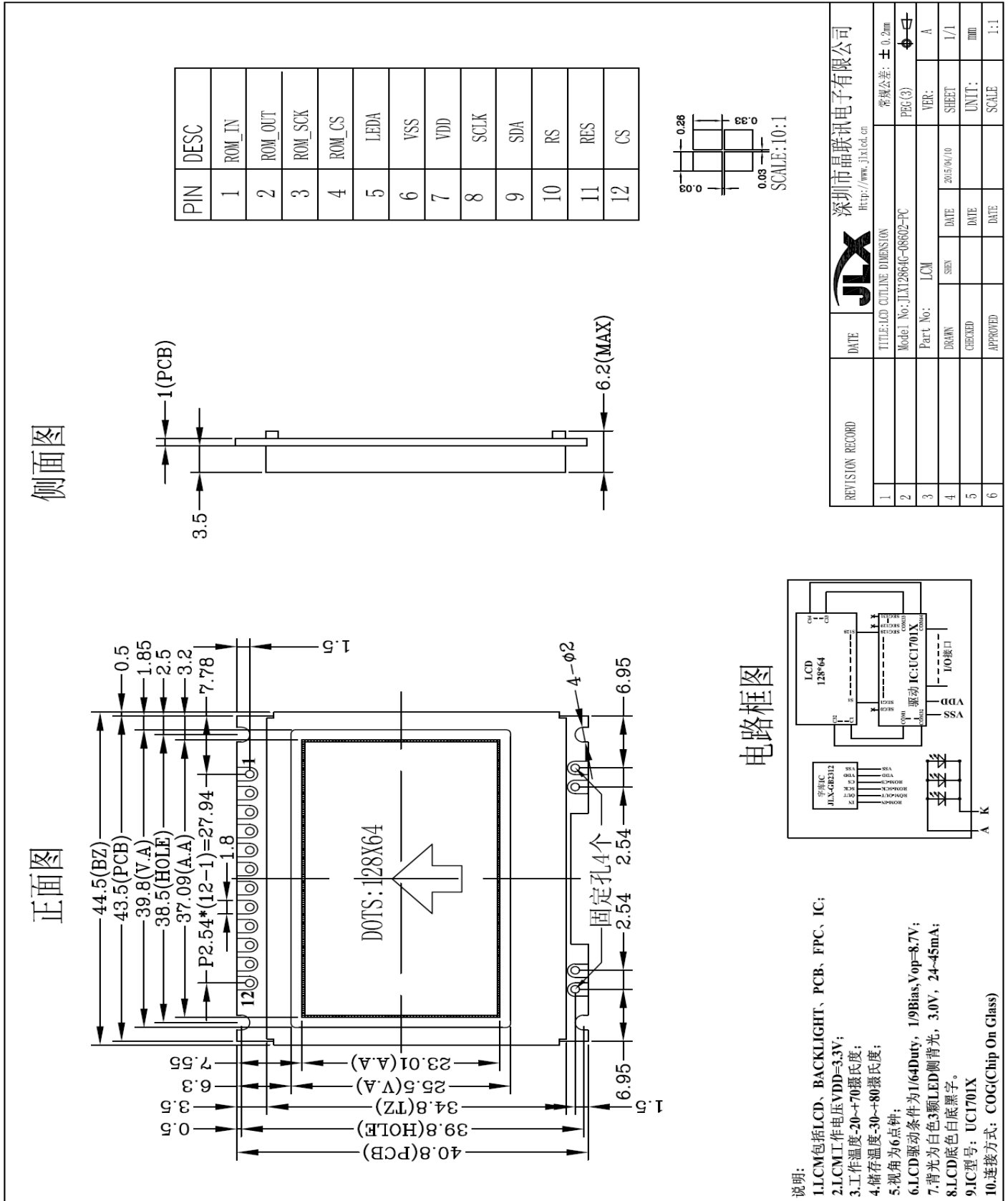
图 1. 外形尺寸
