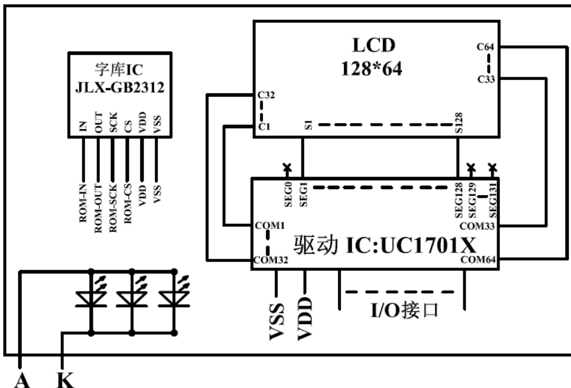
图 2: 电路框图
