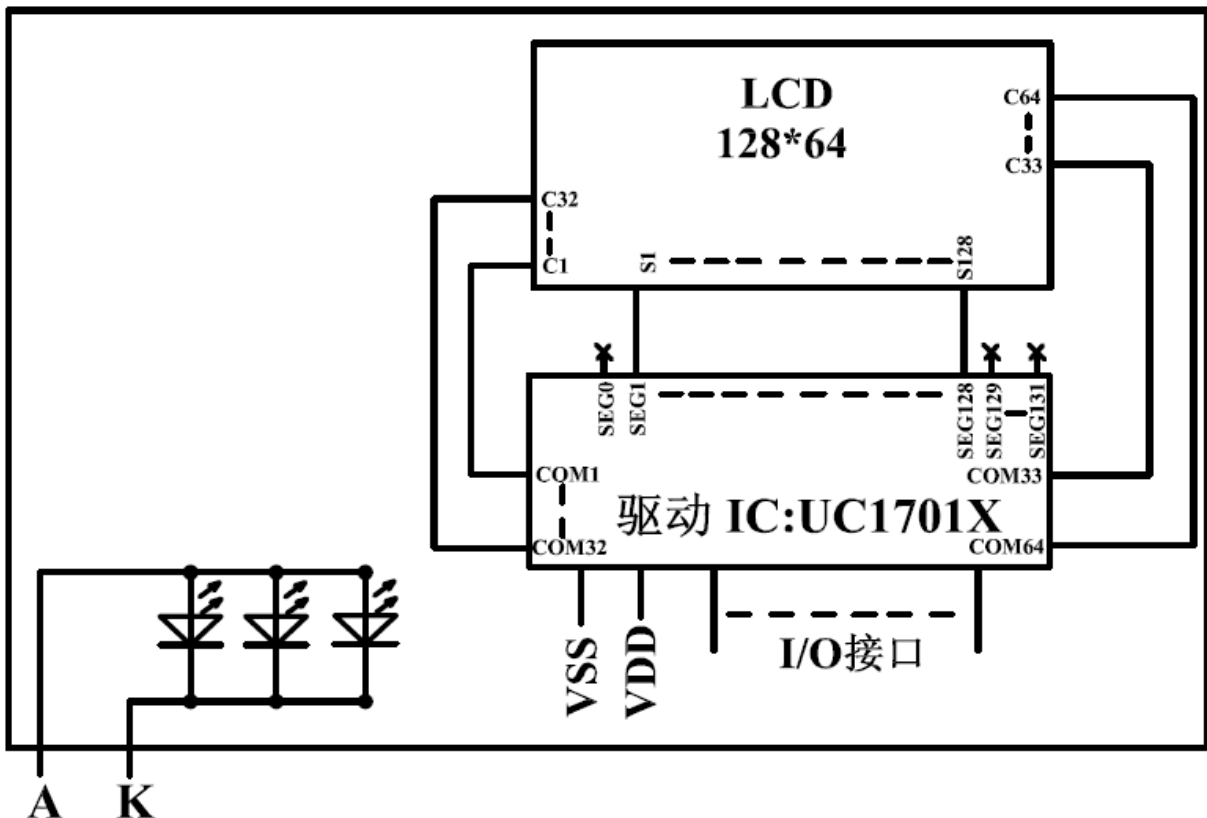
图 2: JLX12864G-08602-PN 图像点阵型液晶模块的电路框图
