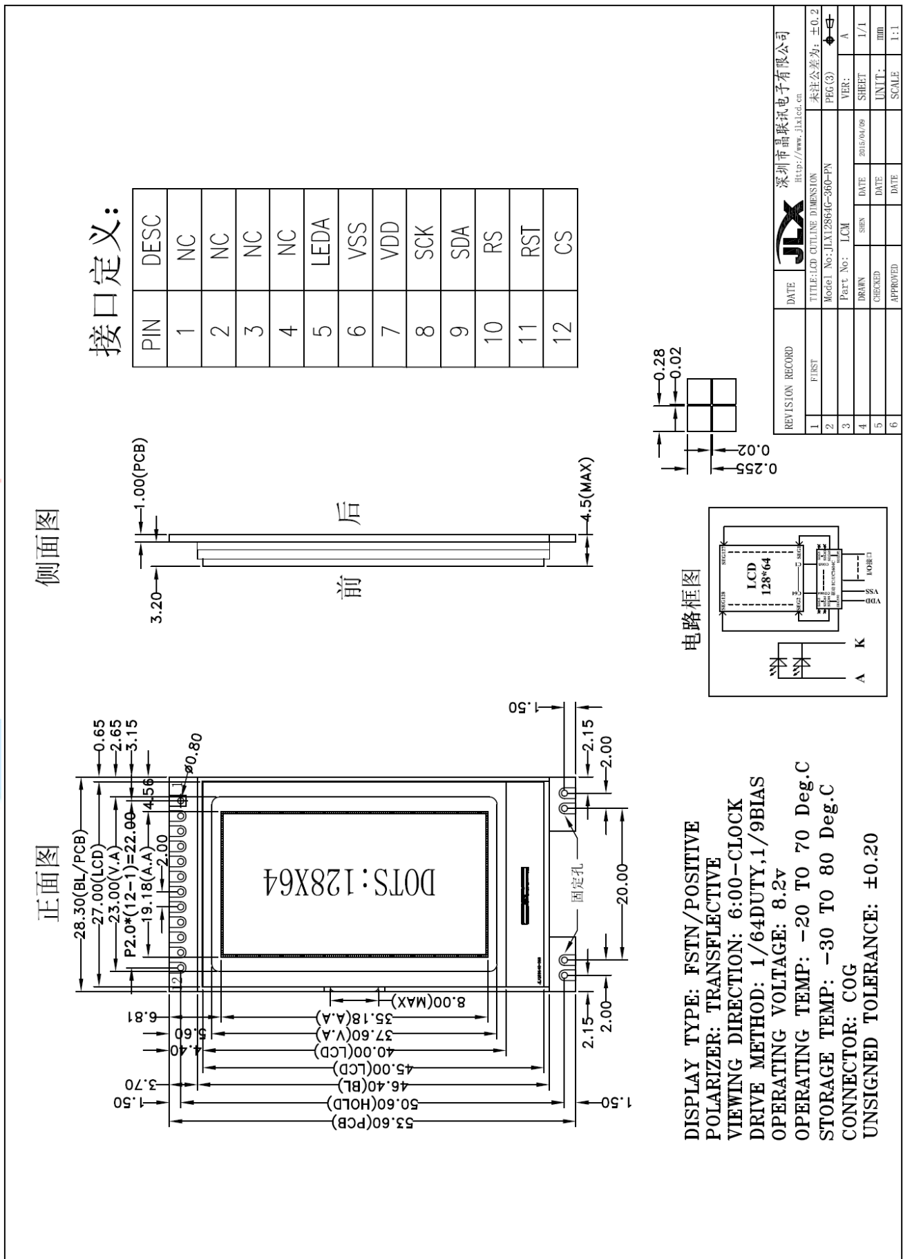
图 1. 外形尺寸
