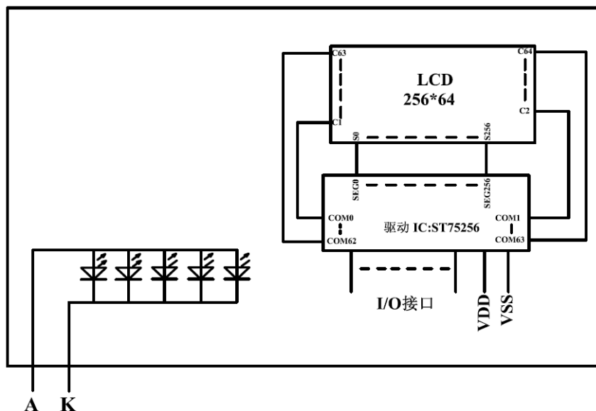
图 2: JLX25664G-251-PN 图像点阵型液晶模块的电路框图
