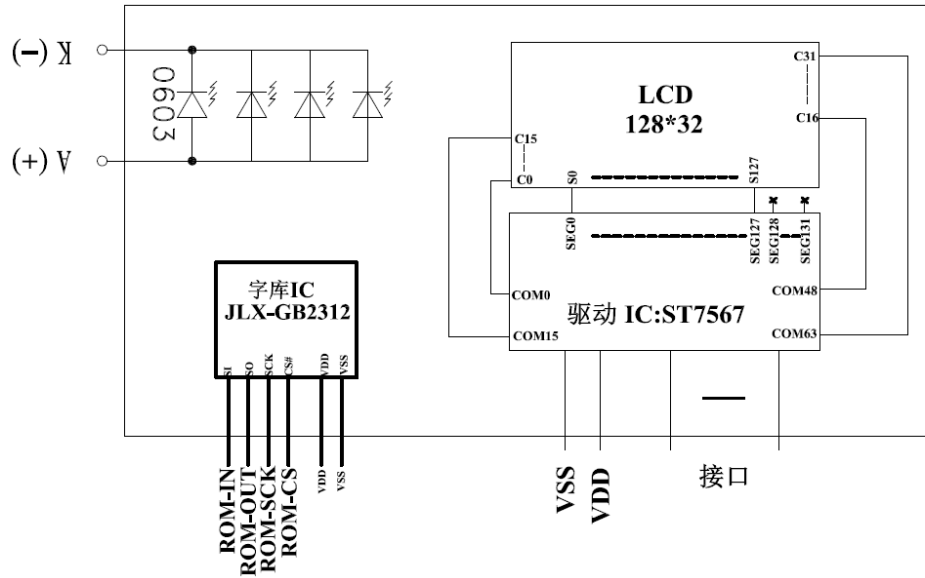
图 2: 电路框图
