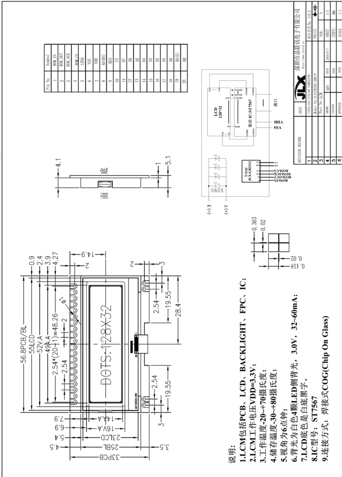
图 1. 外形尺寸
