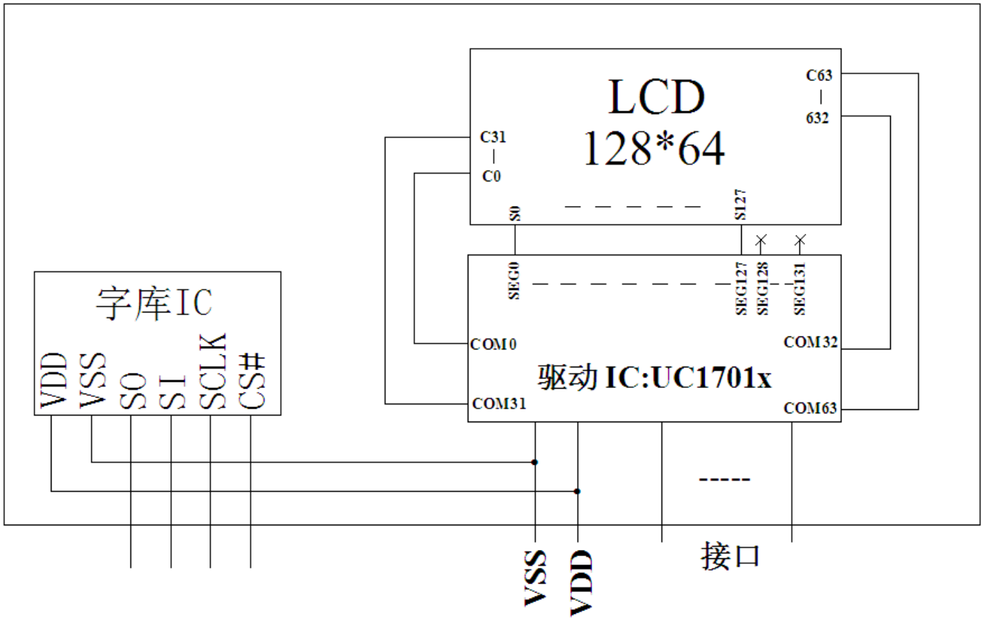
图 2: 电路框图
