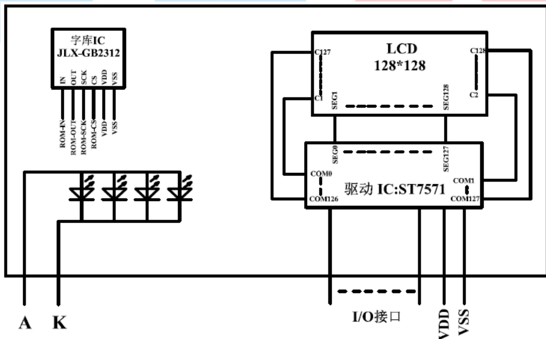
图 2: 电路框图
