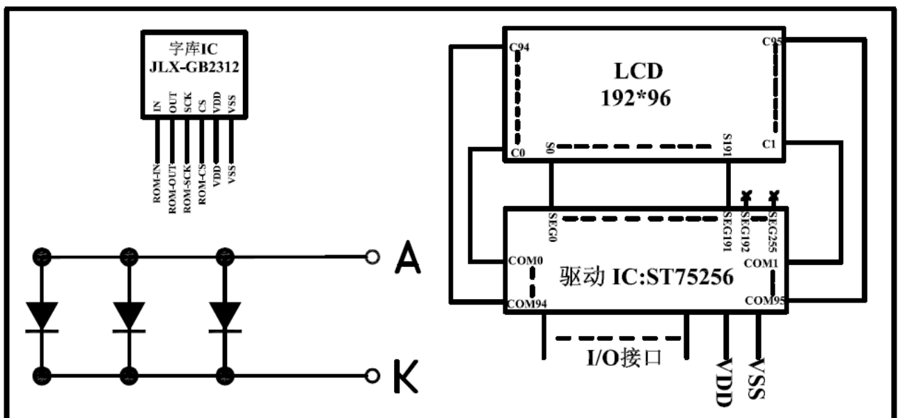
图 2: JLX19296G-690 电路框图
