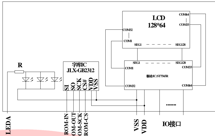
图 2: 电路框图
