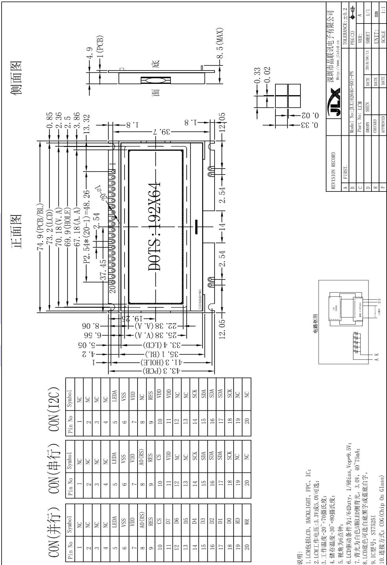
图 1. 外形尺寸
