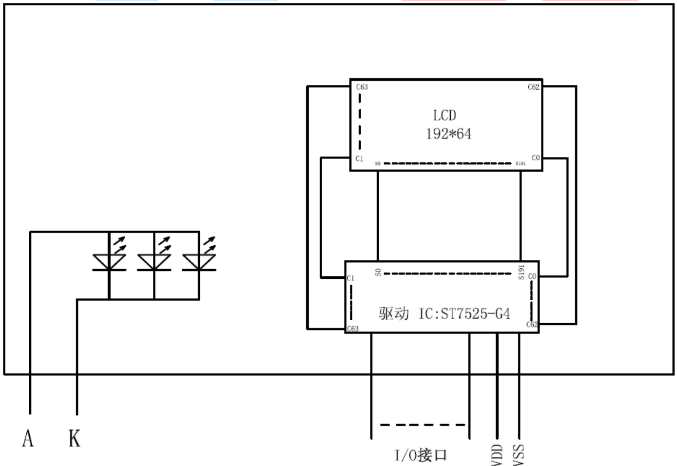
图 2: JLX19264G-740-BN 图像点阵型液晶模块的电路框图
