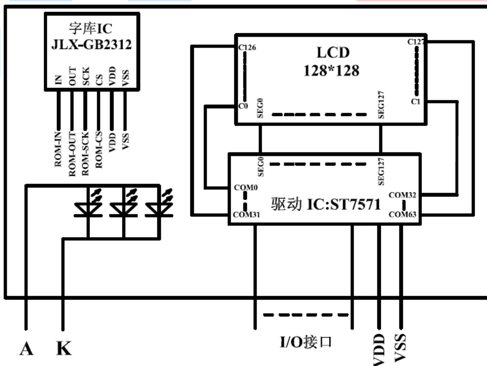
图 2: 电路框图
