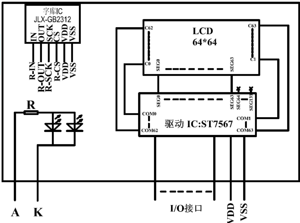
图 2: JLX6464G-720 图像点阵型液晶模块的电路框图
