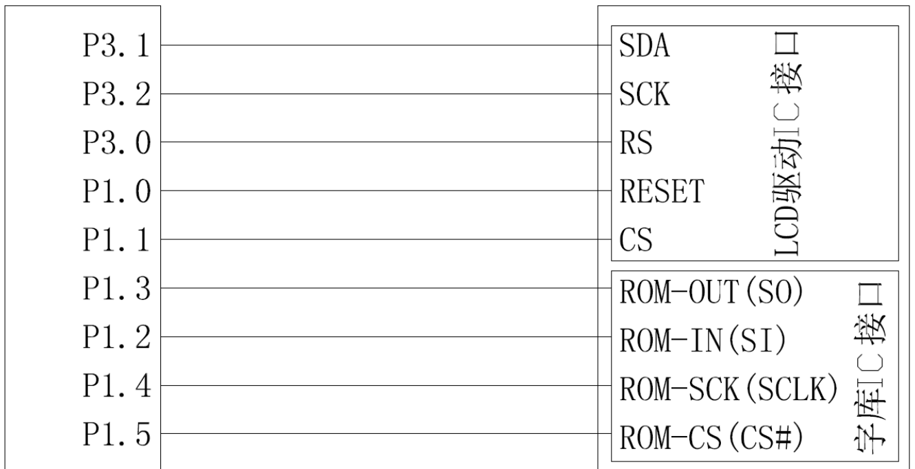
图 5. 串行接口
