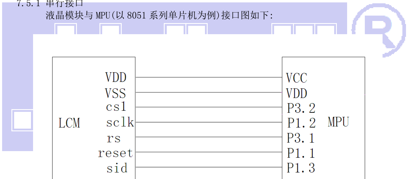
图 9. 串行接口
