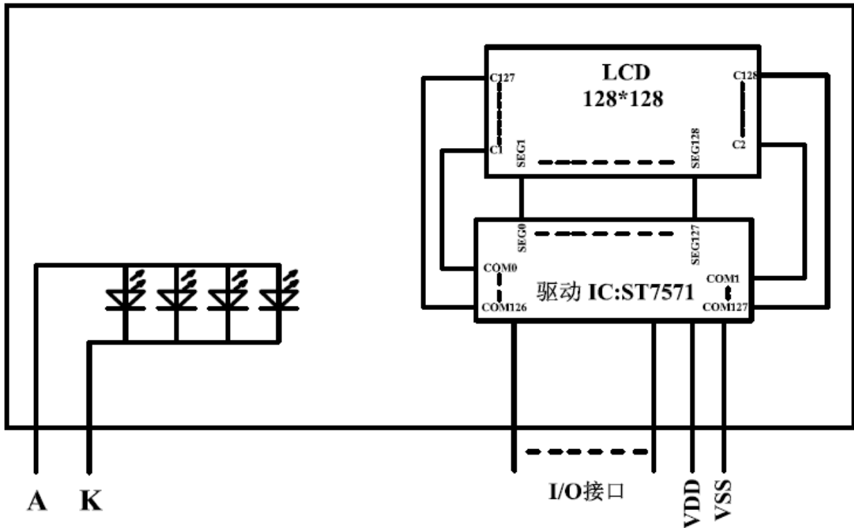
图 2: JLX128128G-610 图像点阵型液晶模块的电路框图
