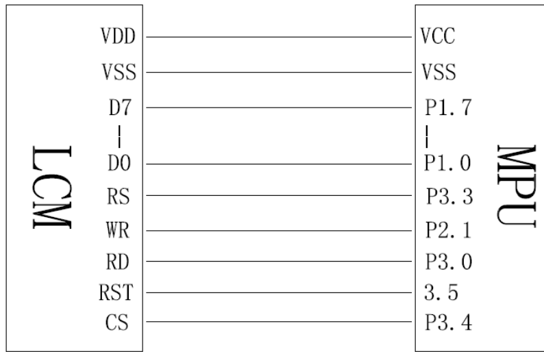
图 8. 并行接口
