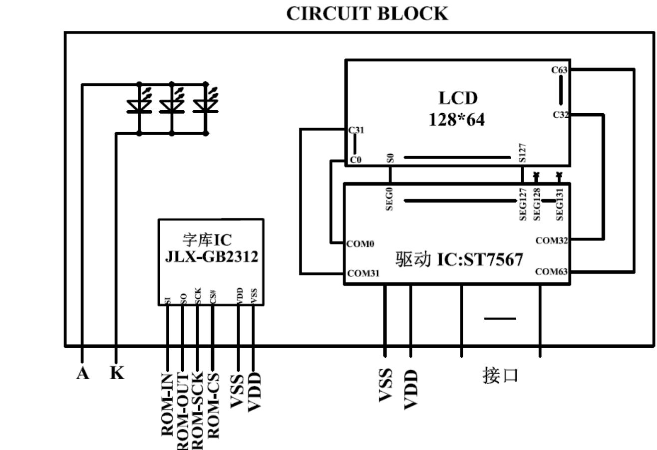
图 2: 电路框图
