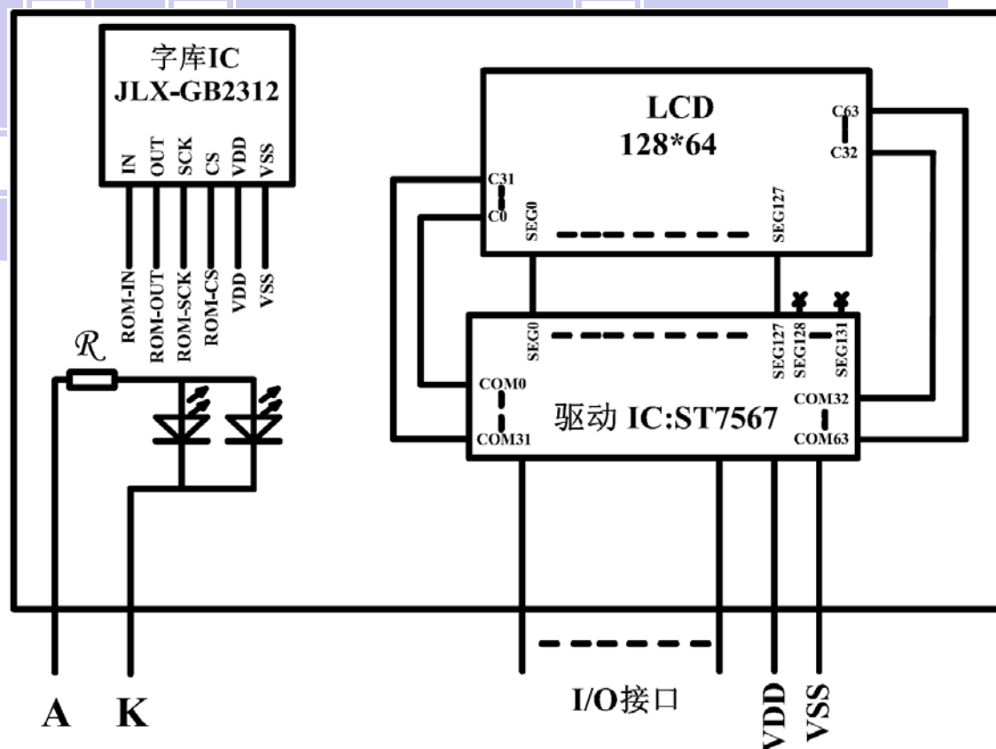
电路框图
