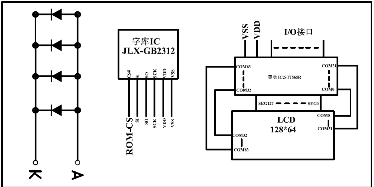
图 2: 电路框图
