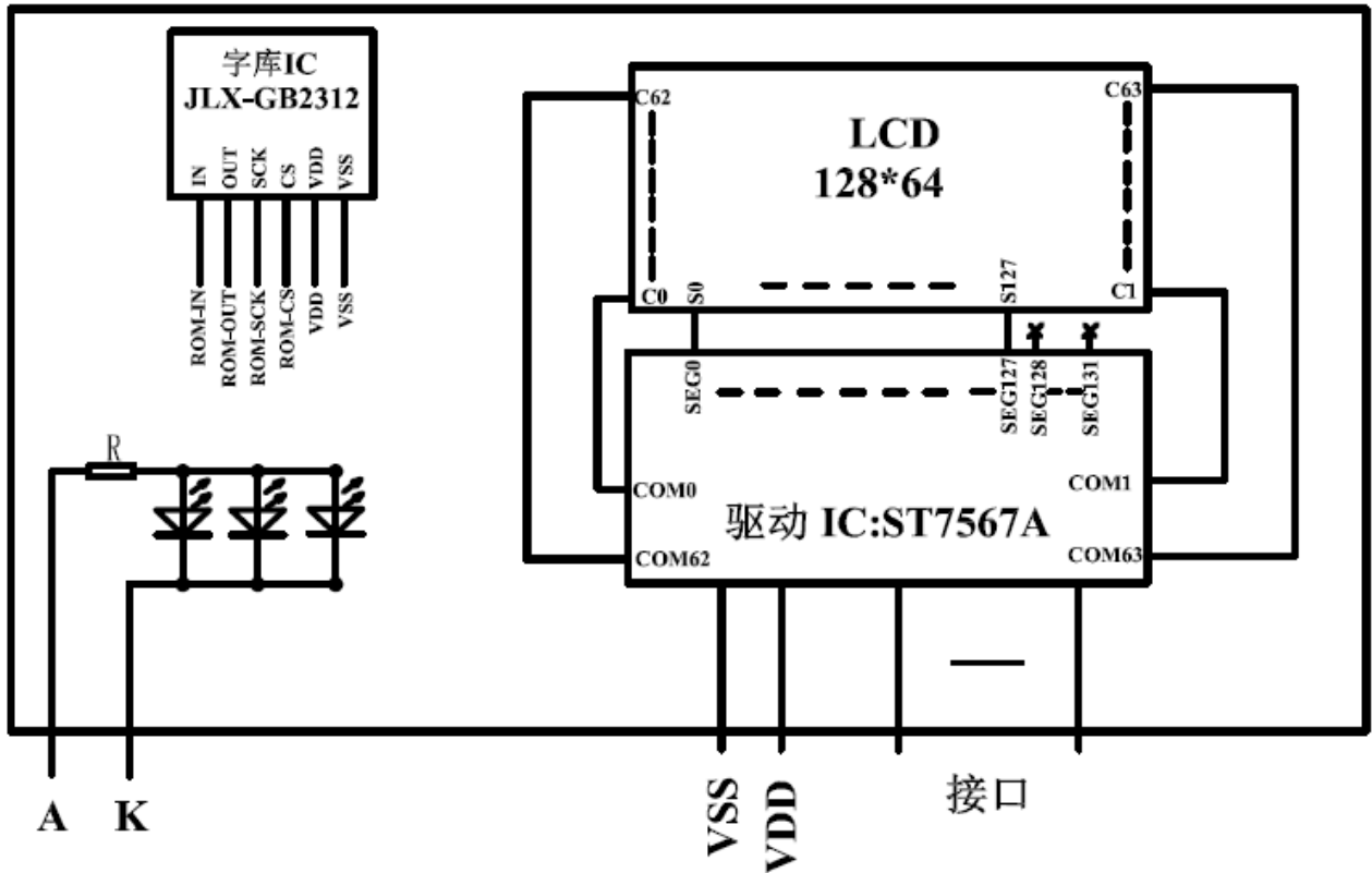
图 2: JLX12864G-755 电路框图
