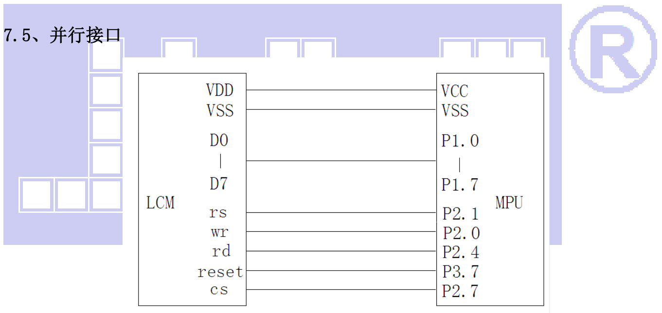
图 9. 并行接口
