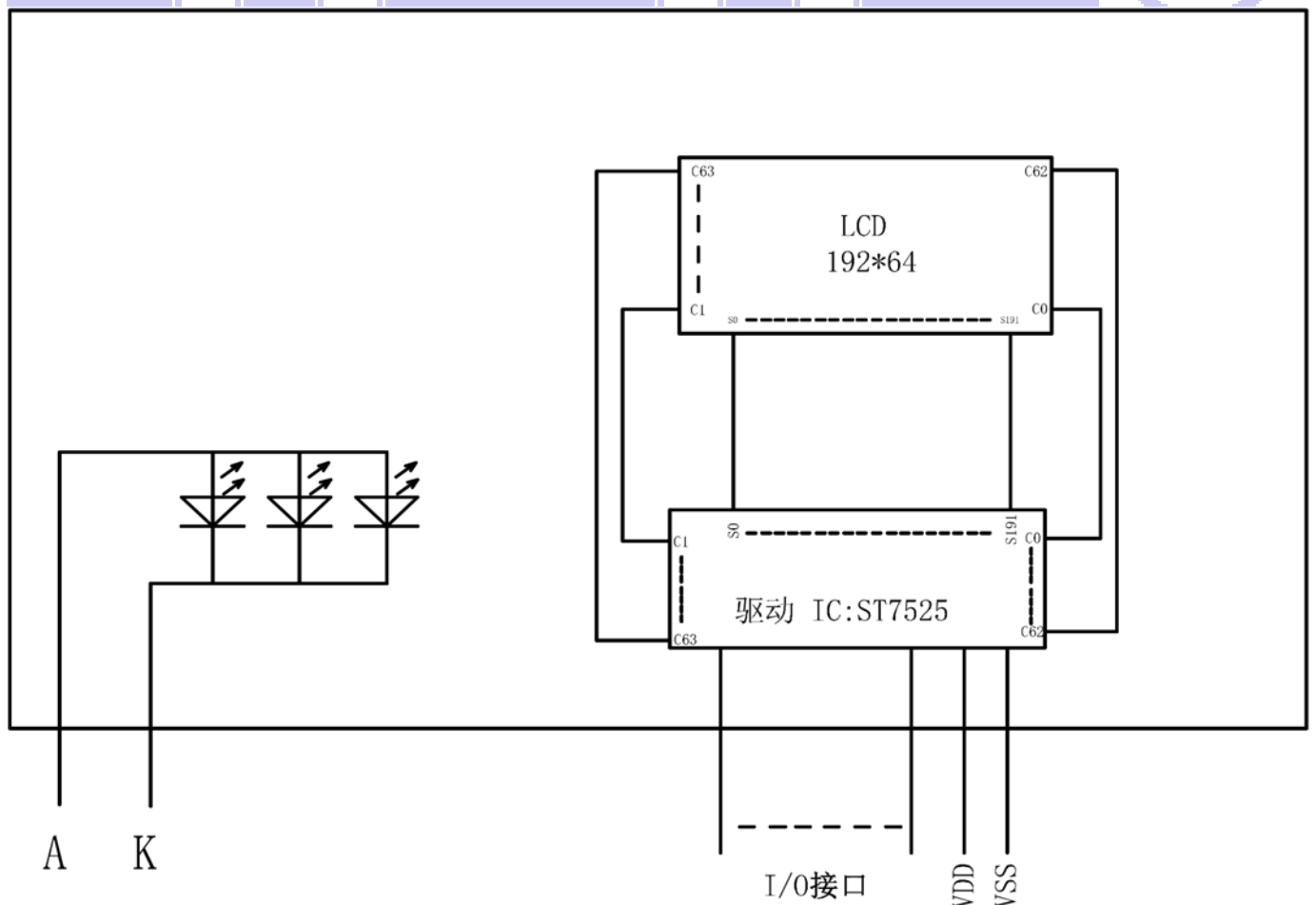
图 2: JLX19264G-74006-BN 图像点阵型液晶模块的电路框图
