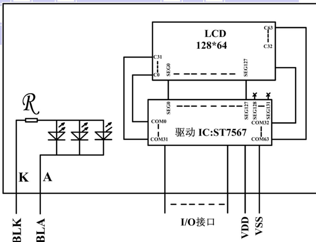
图 2: JLX12864G-33008-PN 图像点阵型液晶模块的电路框图
