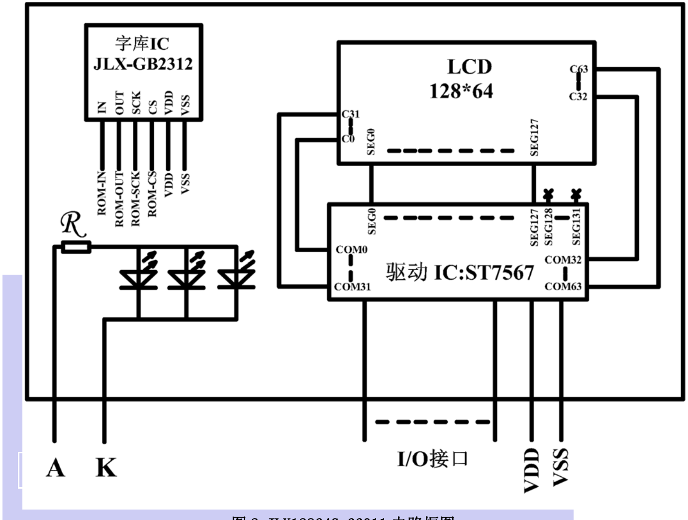
图 2: JLX12864G-66011 电路框图
