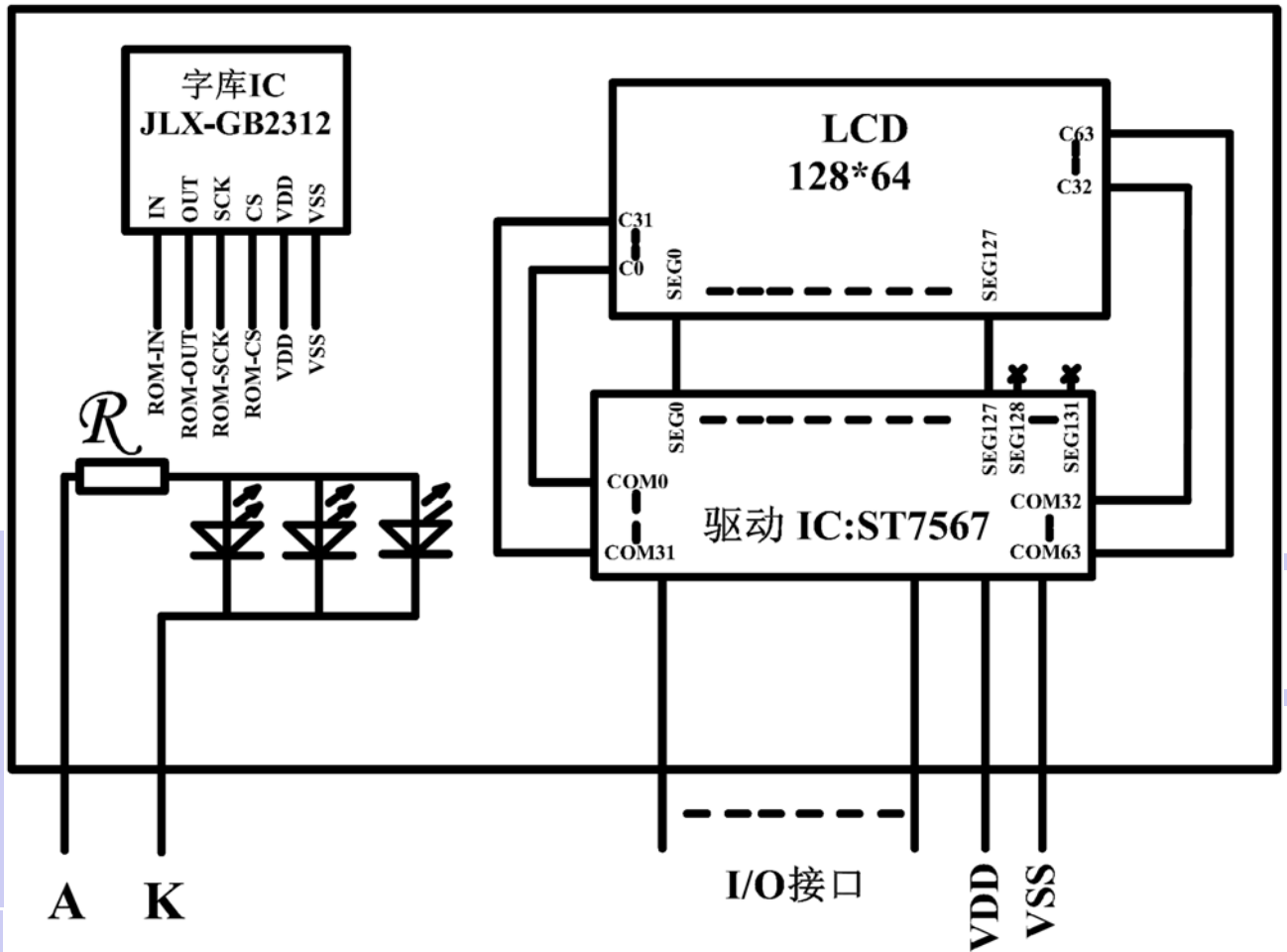
图 2: JLX12864G-66018 电路框图
