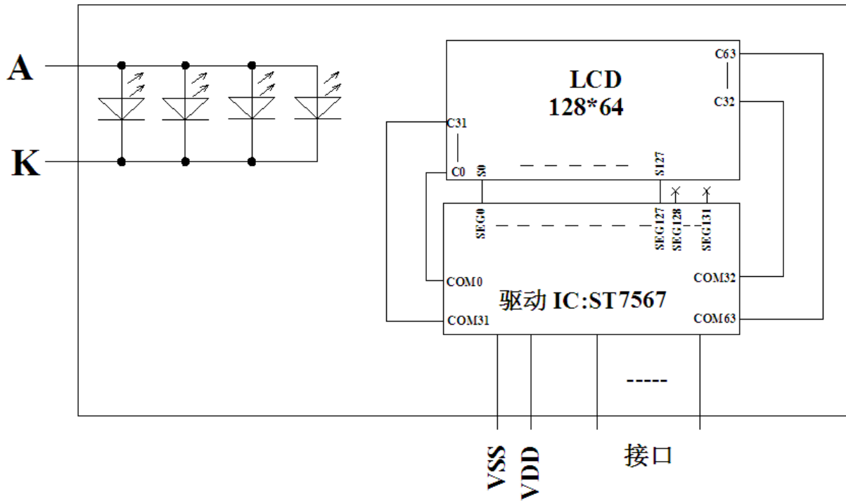
图 2: JLX12864G-9309-PN 图像点阵型液晶模块的电路框图
