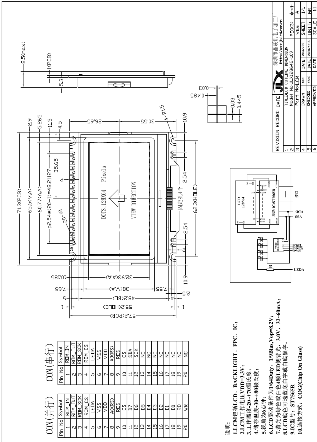
图 1. 外形尺寸
