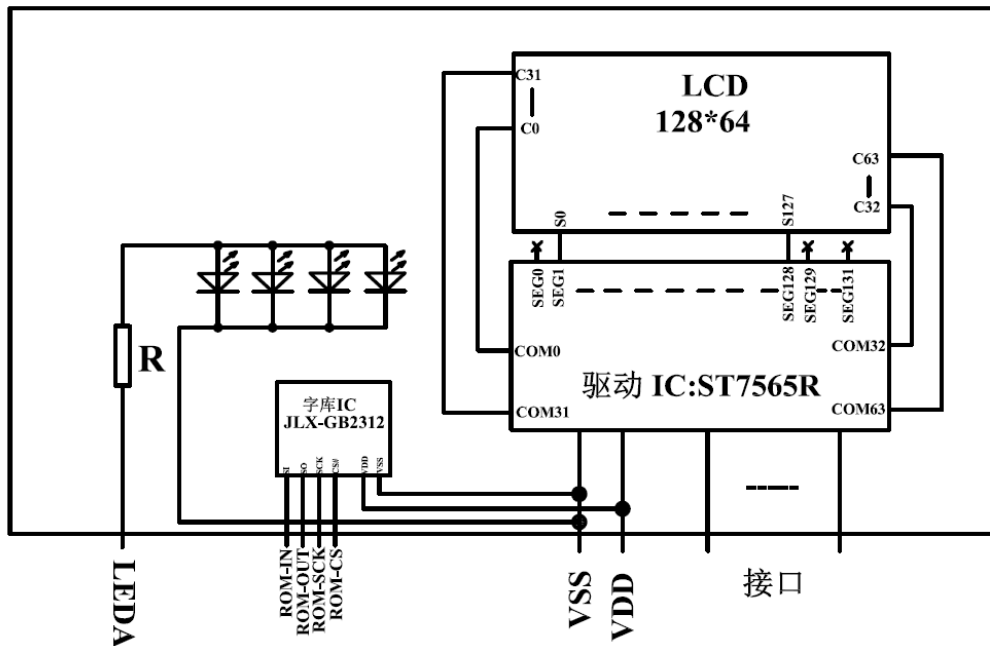
图 2: 电路框图
