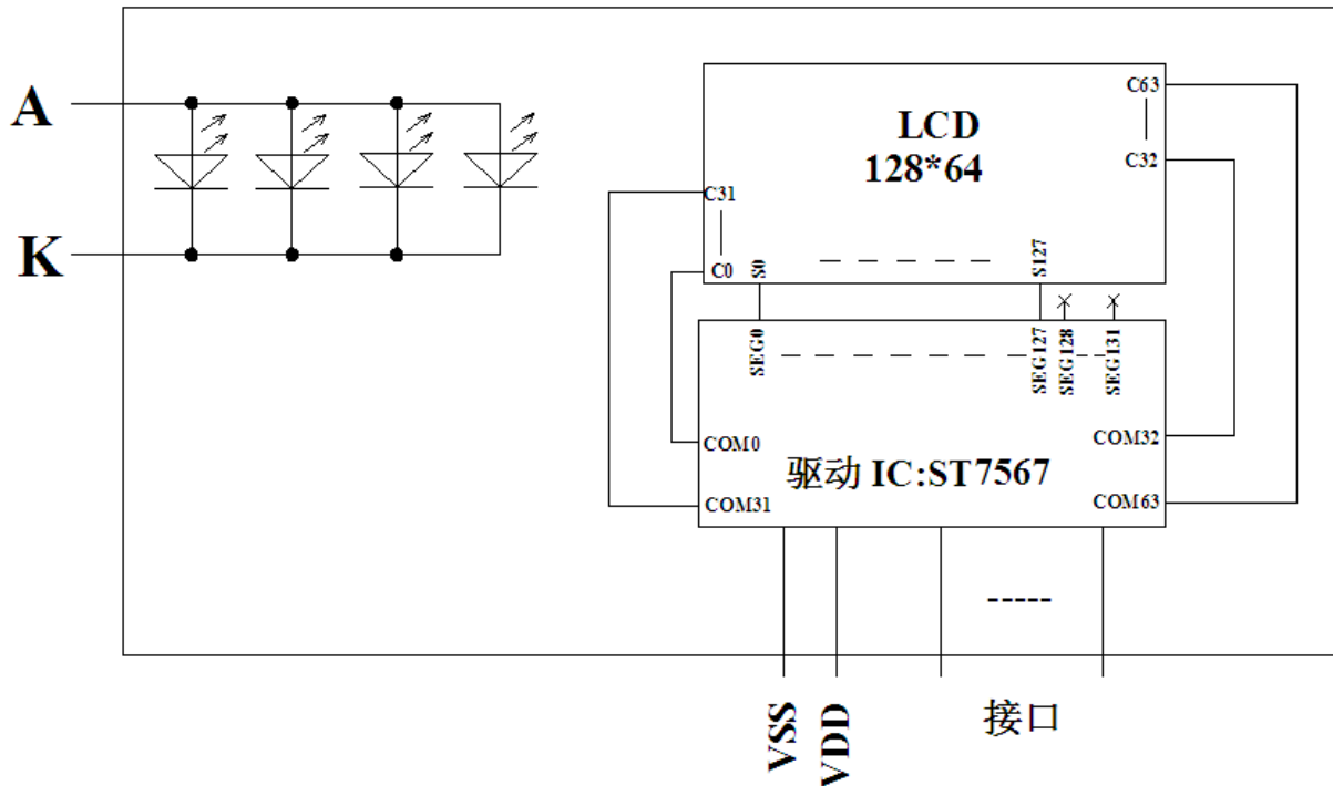
图 2: JLX12864G-9309-PN 图像点阵型液晶模块的电路框图
