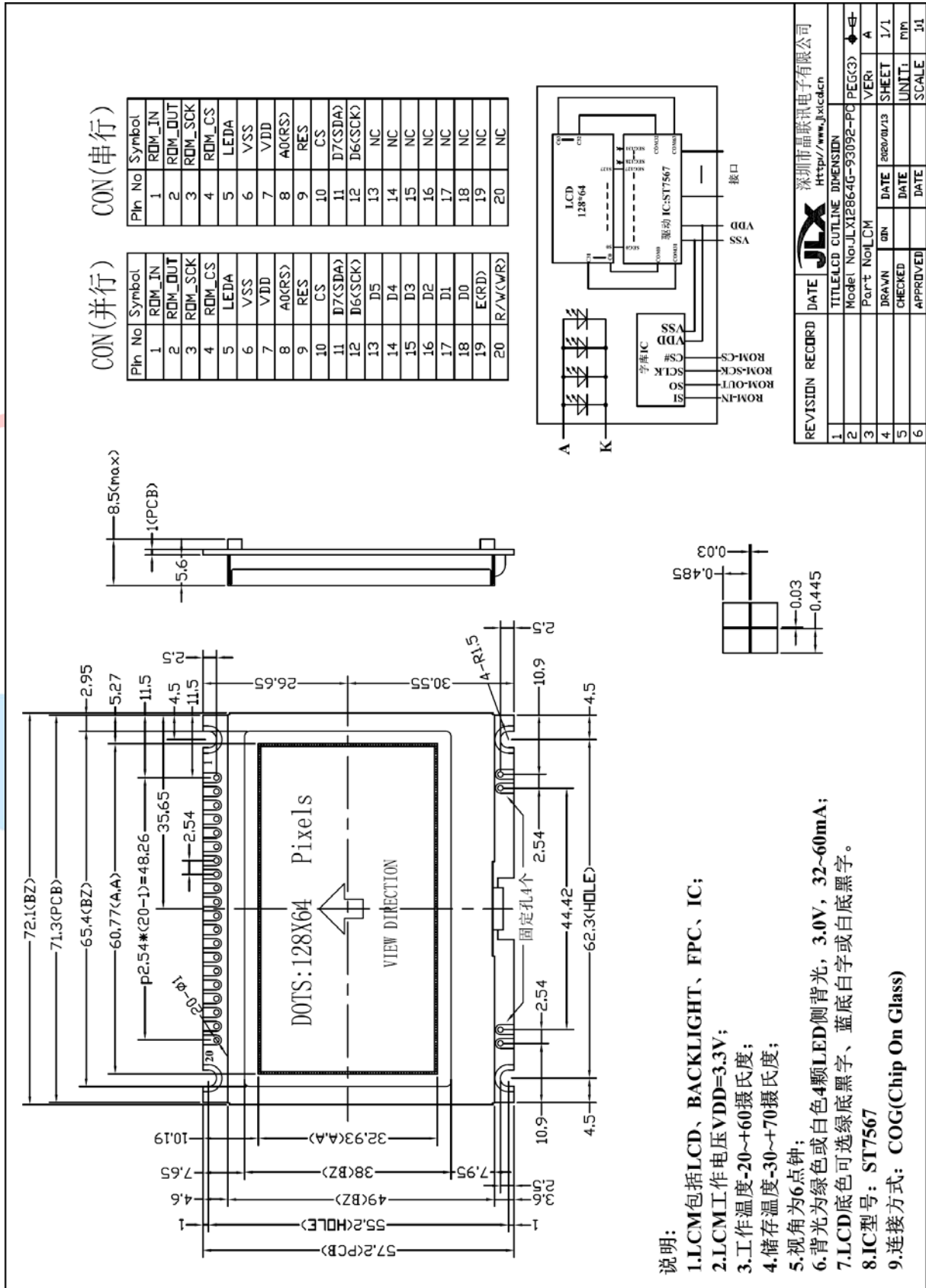
图 1. 外形尺寸
