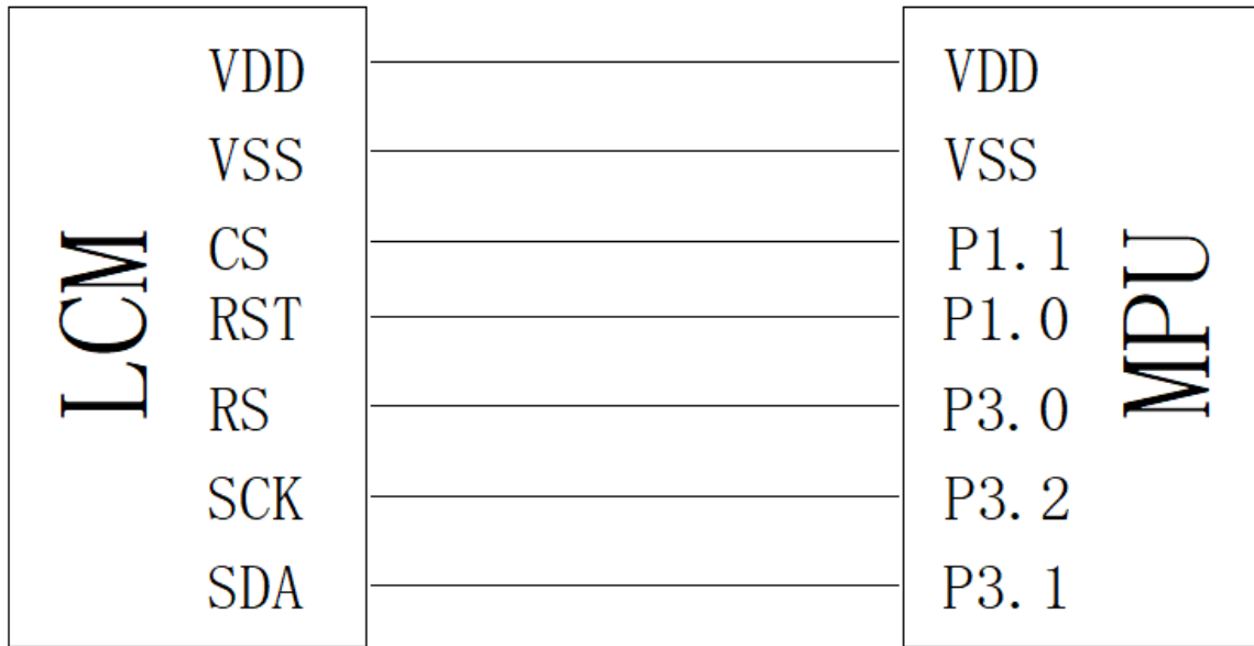
图 8. 串行接口
