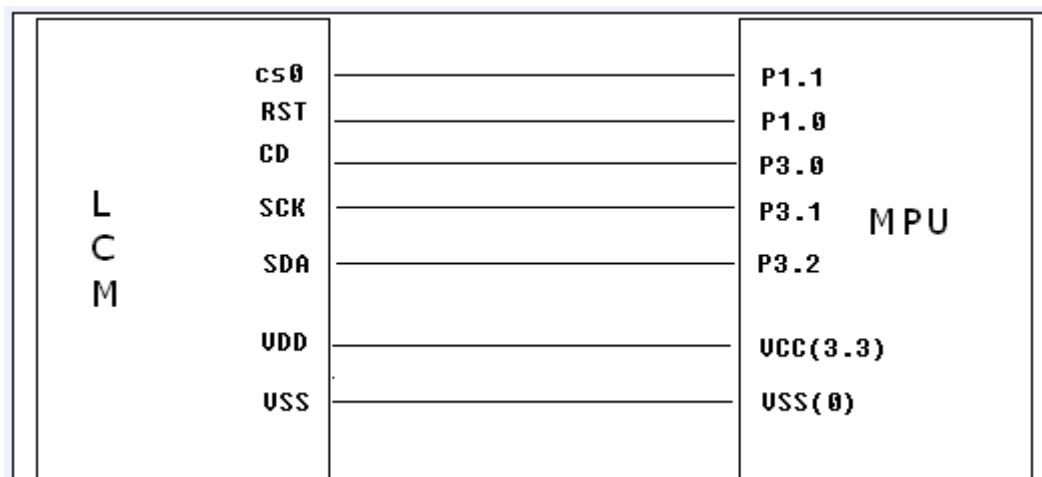
图 4. 串行接口
