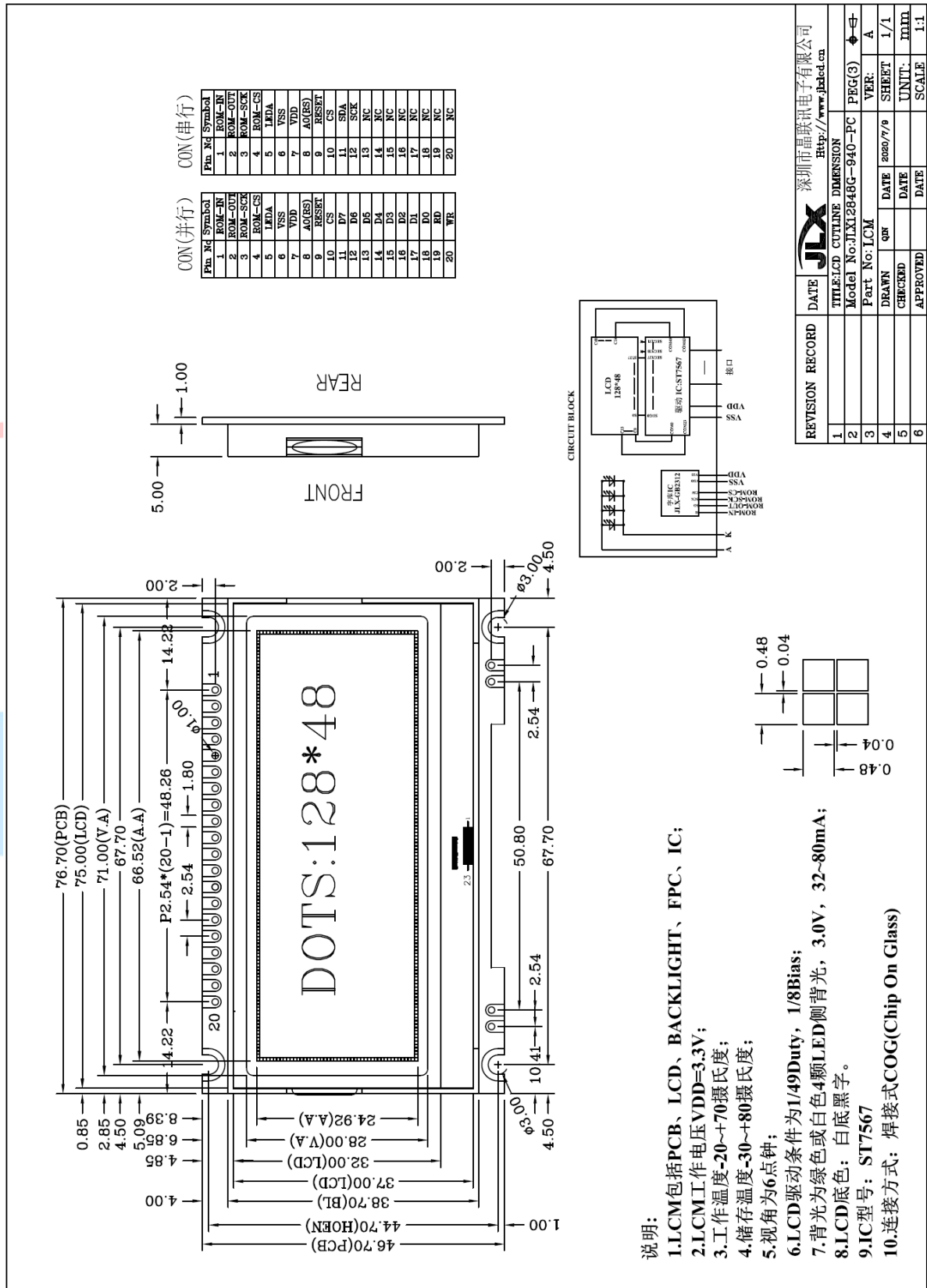
图 1. 外形尺寸
