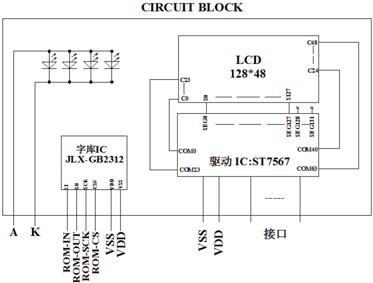
图 2: 电路框图
