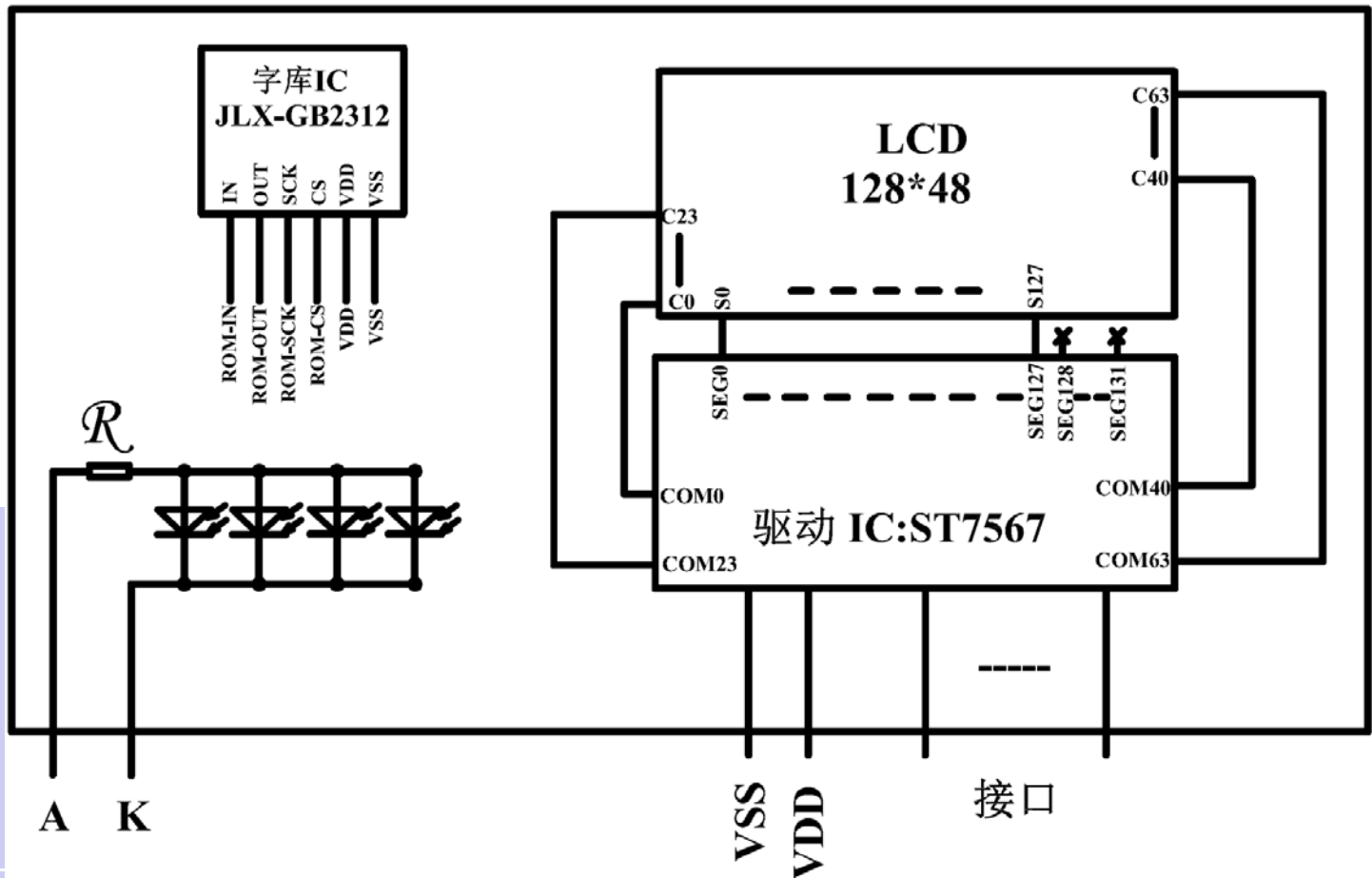
图 2: JLX12848G-941 电路框图
