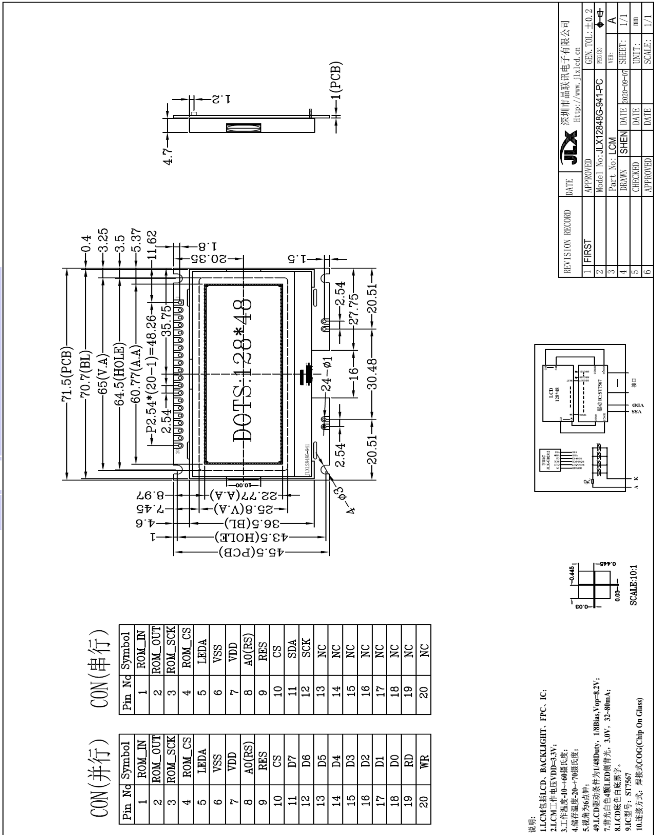
图 1. 外形尺寸
