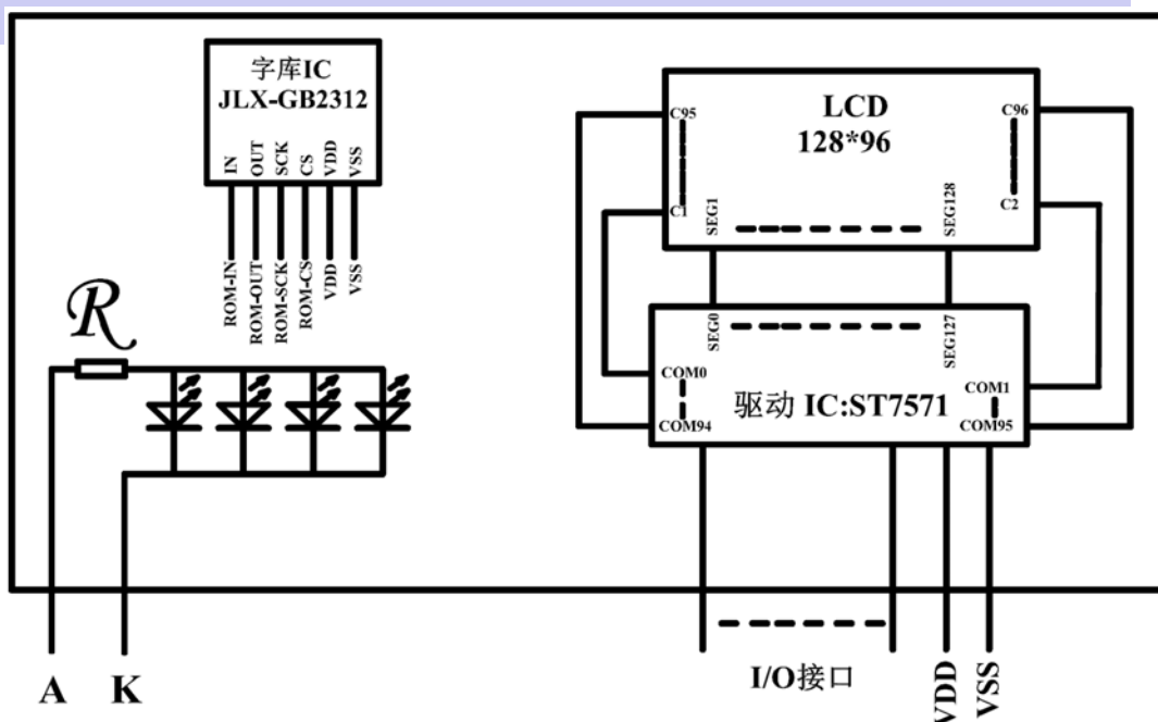
图 2: 电路框图
