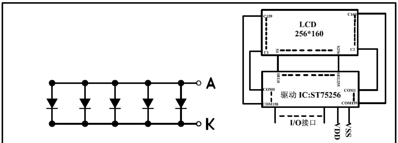
图 2: JLX256160G-910-BN 图像点阵型液晶模块的电路框图
