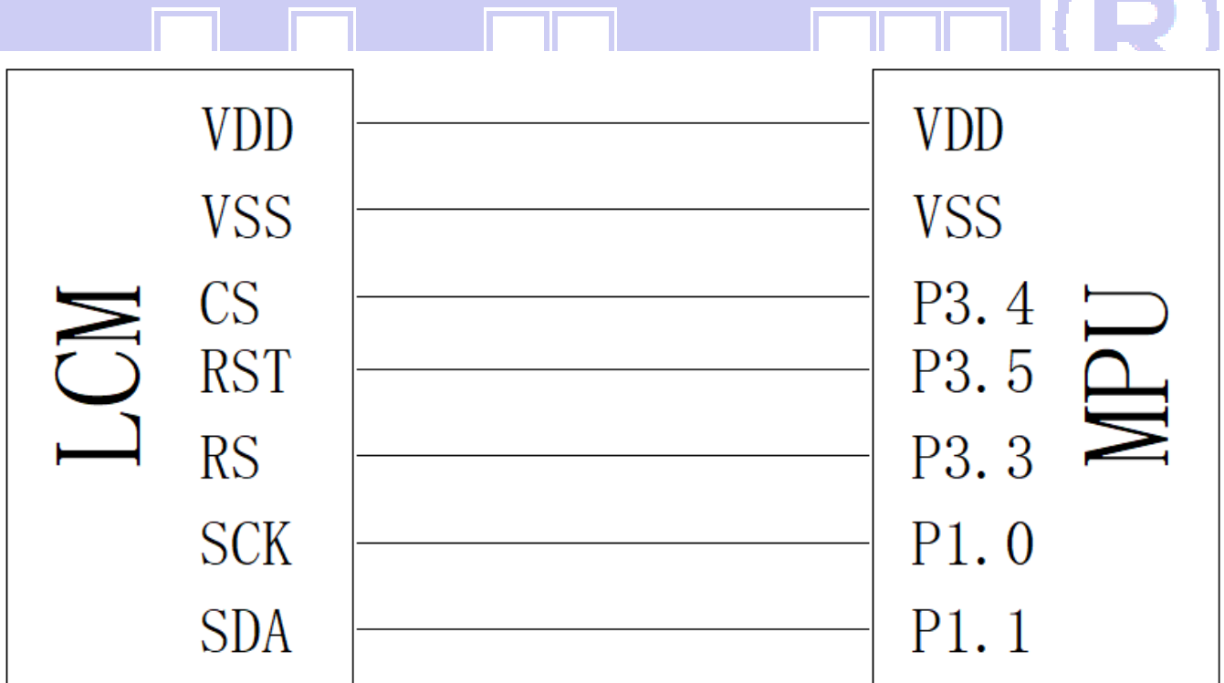
图 9. 串行接口
