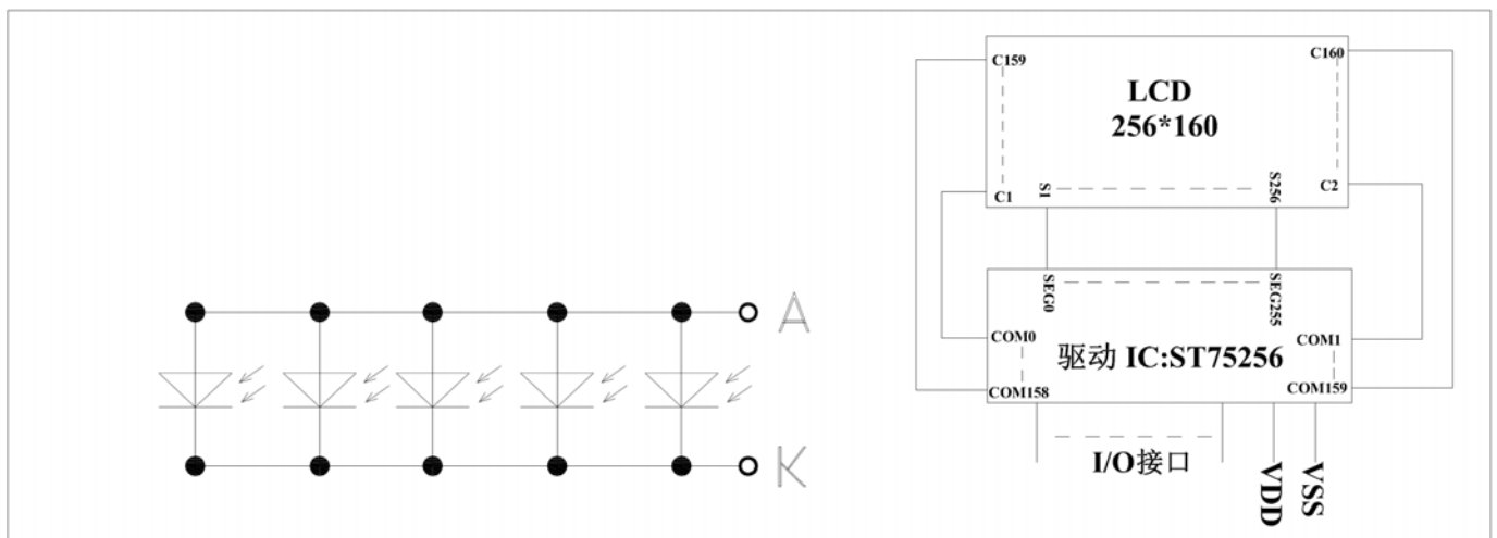
图 2: JLX256160G-91006-BN 图像点阵型液晶模块的电路框图
