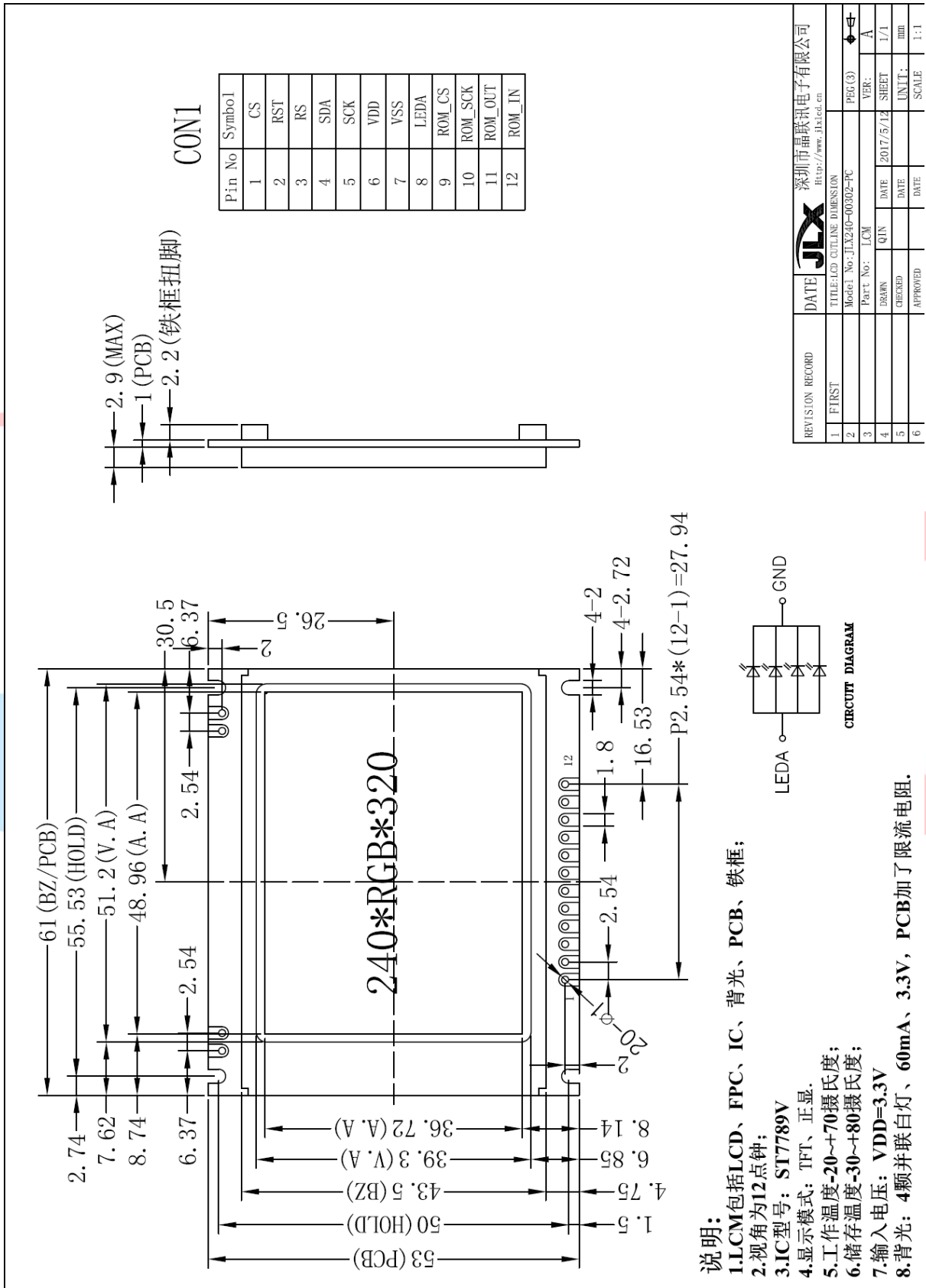
图 1. 外形尺寸
