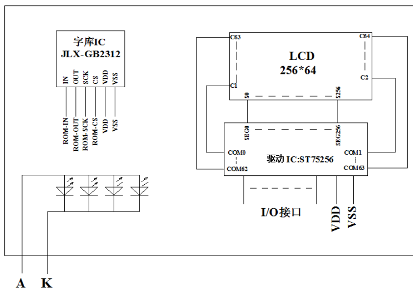
图 2: JLX25664G-960-PC 电路框图
