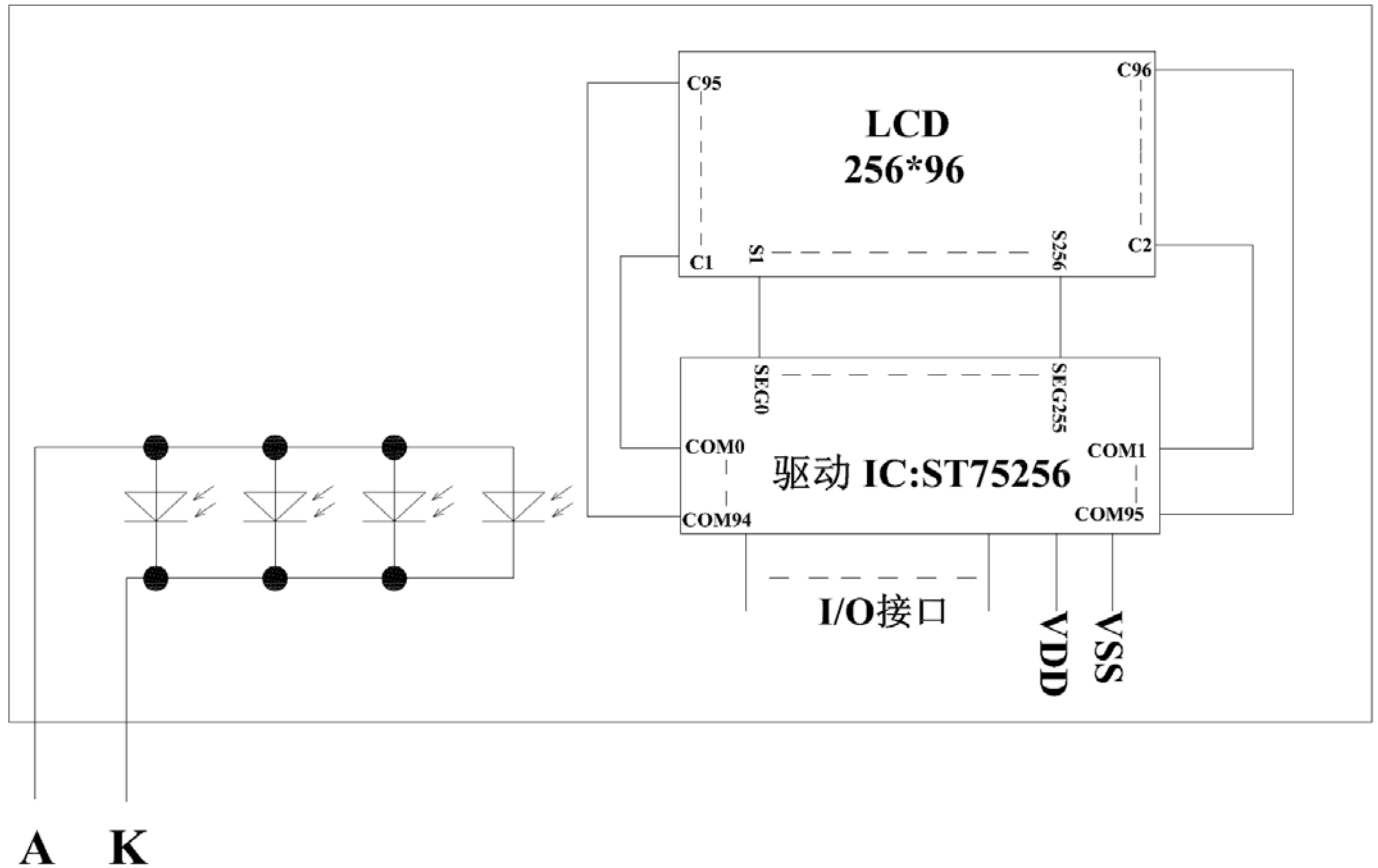
图 2: JLX25696G-967-BN 图像点阵型液晶模块的电路框图
