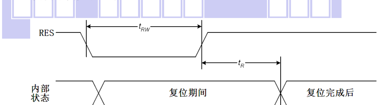
图 7：电源启动后复位的时序
