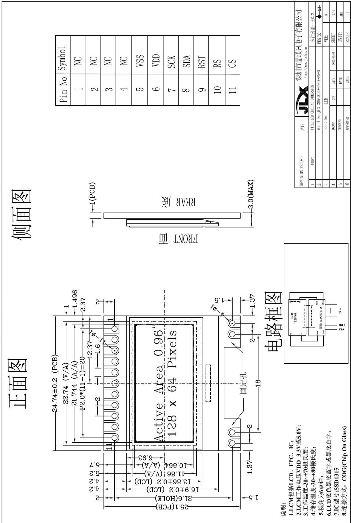
图 1. 模块外形尺寸
