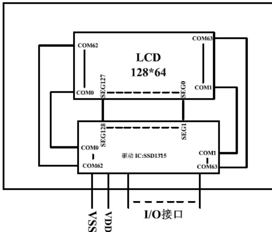
图 2. JLX12864OLED-096X
