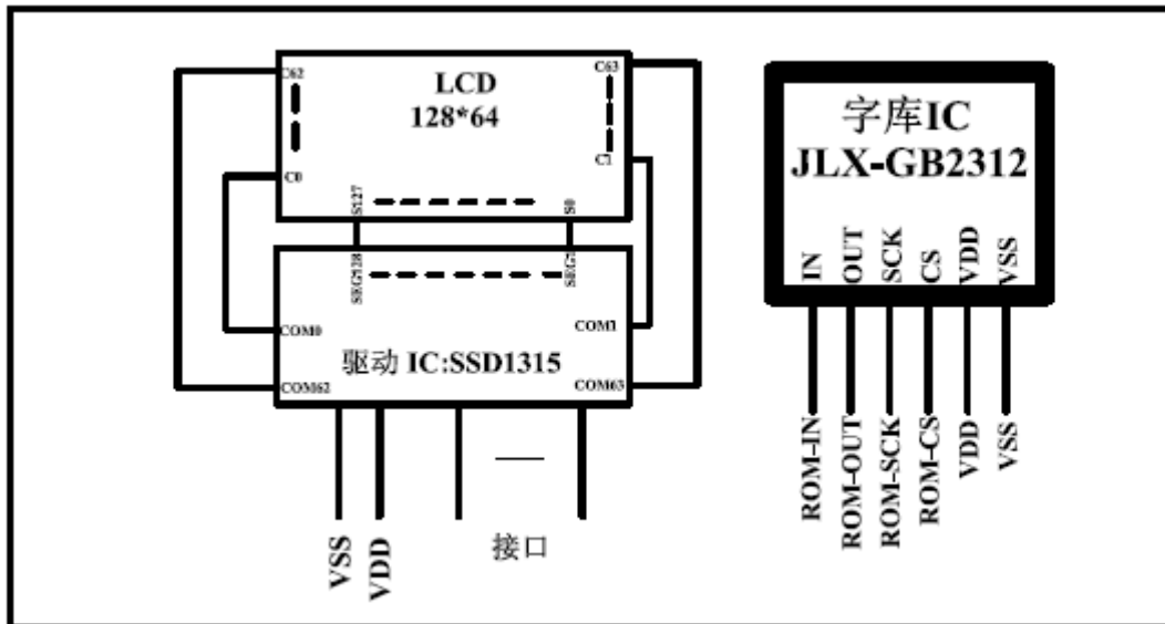
图 2. JLX12864OLED-096X-PC-11C
