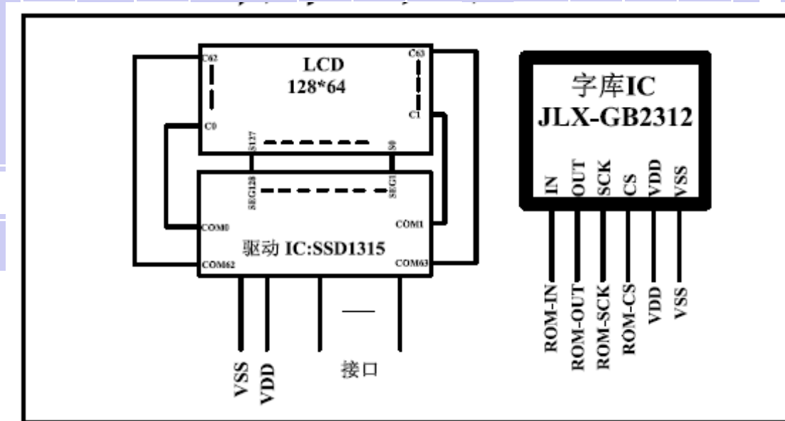
图 2. JLX12864OLED-096X-PC-IIC
