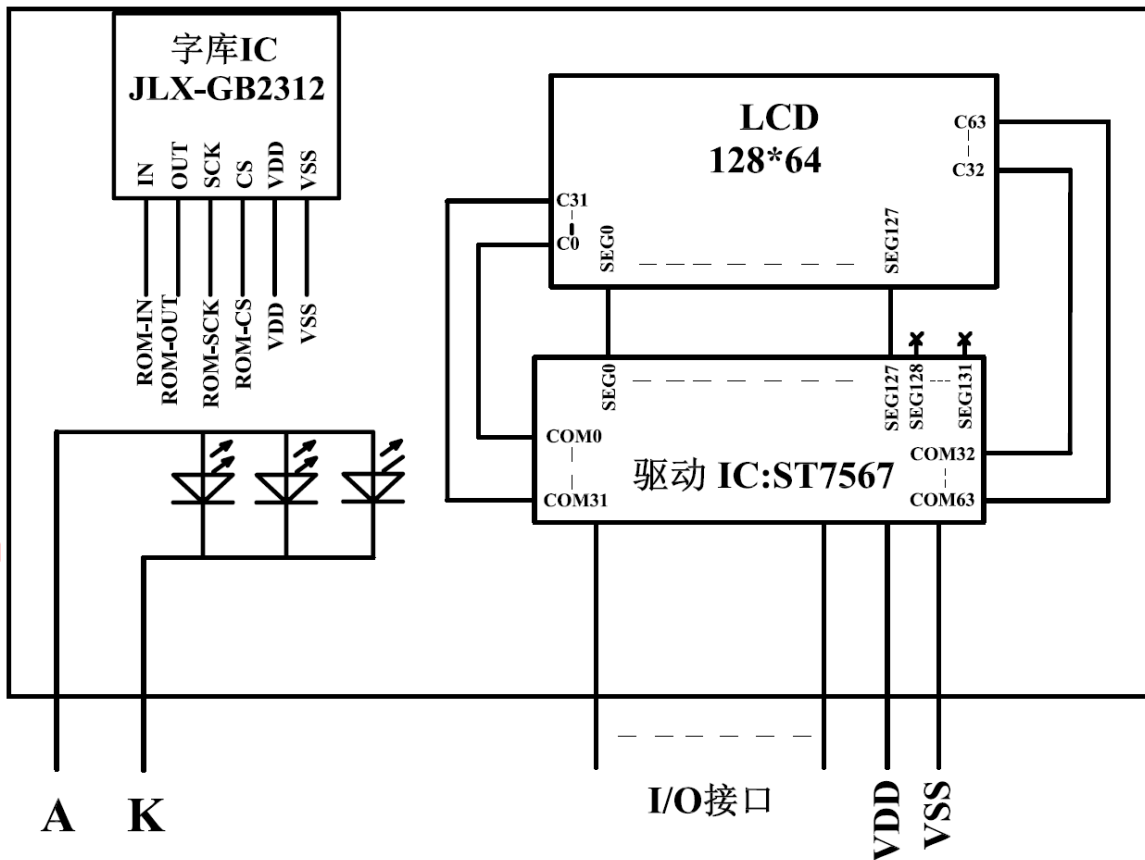
图 2: JLX12864G-09505 电路框图
