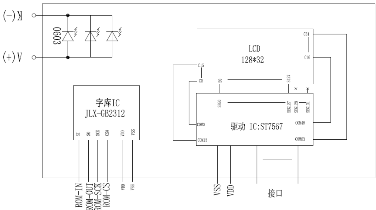
图 2: 电路框图
