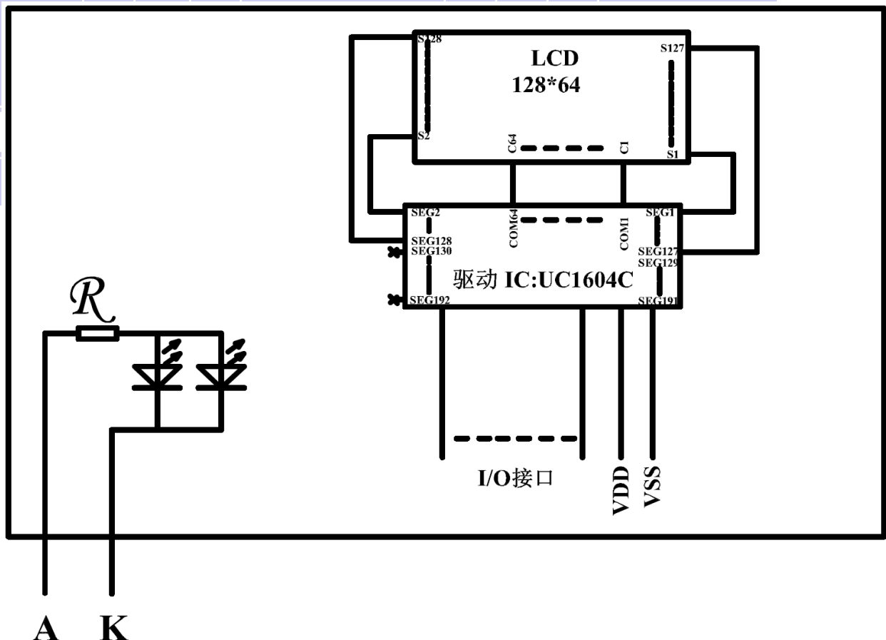
图 2: JLX12864G-936 图像点阵型液晶模块的电路框图
