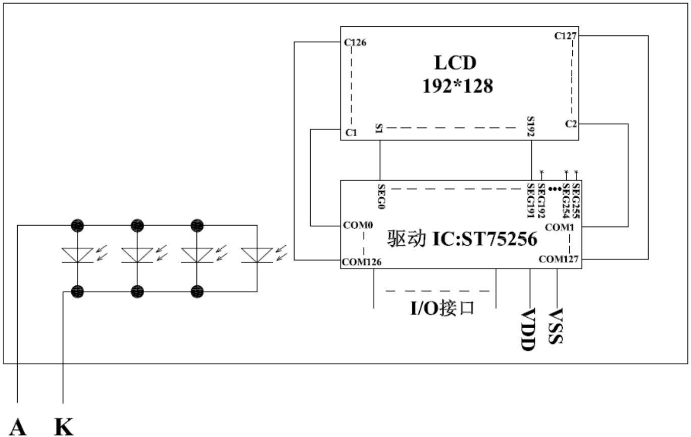
图 2: JLX192128G-970-BN 图像点阵型液晶模块的电路框图
