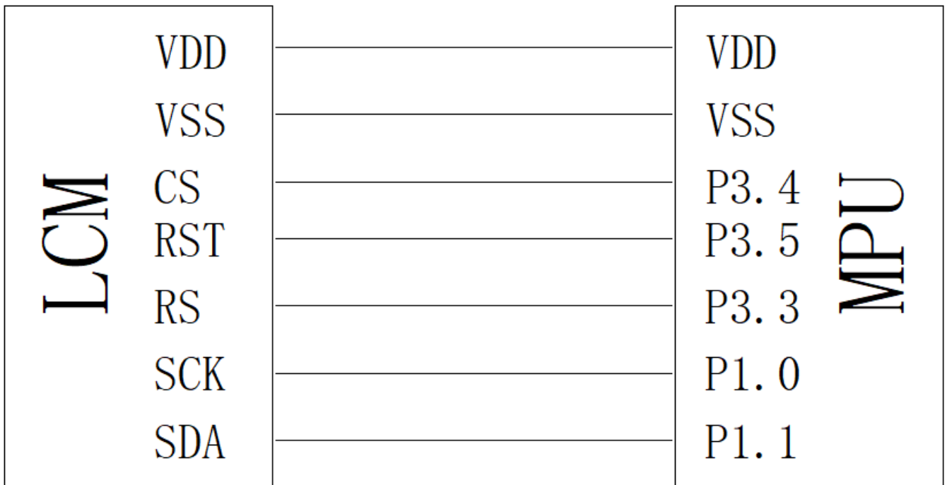
图 9. 串行接口
